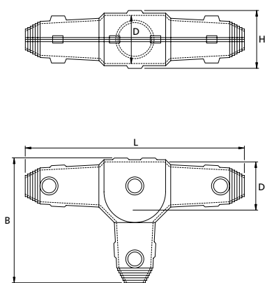
Afmetingen T1
