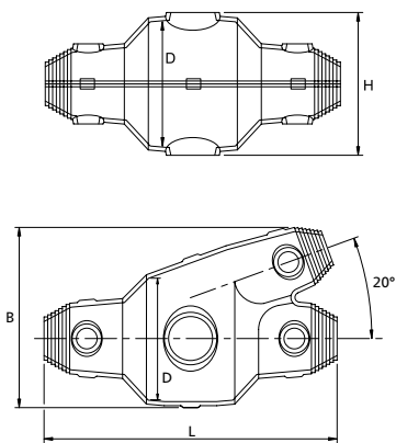
Afmetingen Y1
