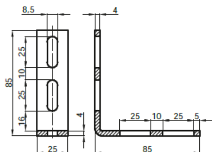
RECHTE 90° HOEK
