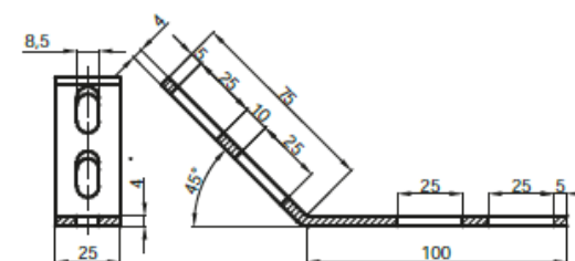
45° hoek
