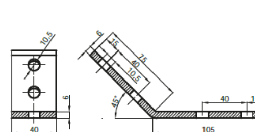
45° hoek
