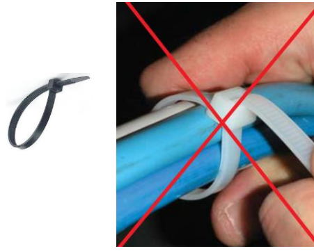
3. Vermijd het om in een scherpe hoek de kabelbinder "over de kop" aan te trekken. Het maakt de verbinding niet sterker.
